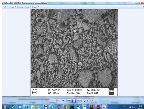
rasm 3. Avtomobil yo'l qoplamalari yeyilishi natijasida hosil bo'lgan qattiq zarralar
