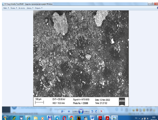
rasm 1. Tormoz ustquymalarining yeyilishi natijasida hosil bo'lgan qattiq zarralar
