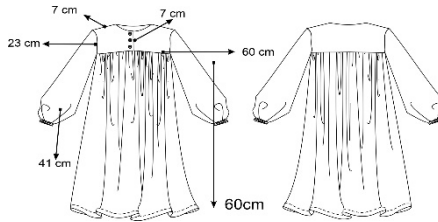
Çizim 6. Elbise Ön-Arka
