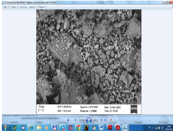
rasm 2. Shinalar yeyilishidan hosil bo'lgan qattiq zarralar
