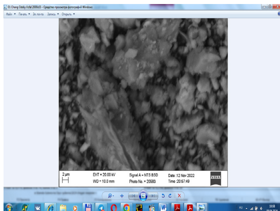
rasm 4. Avtomobil yo'l qoplamalari yeyilishi natijasida qayta to'plangan yo'l changi
